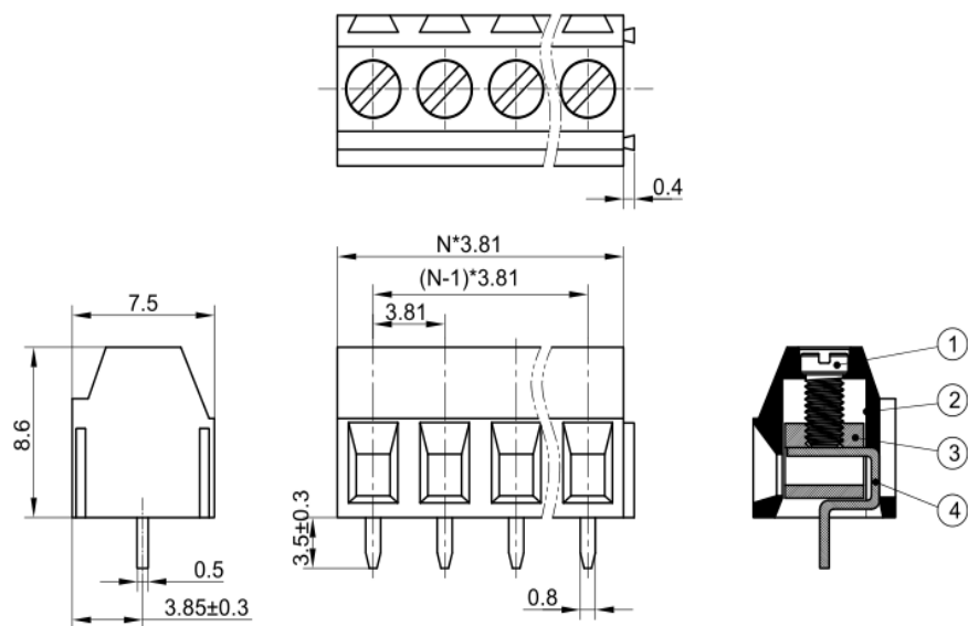
尺寸图
