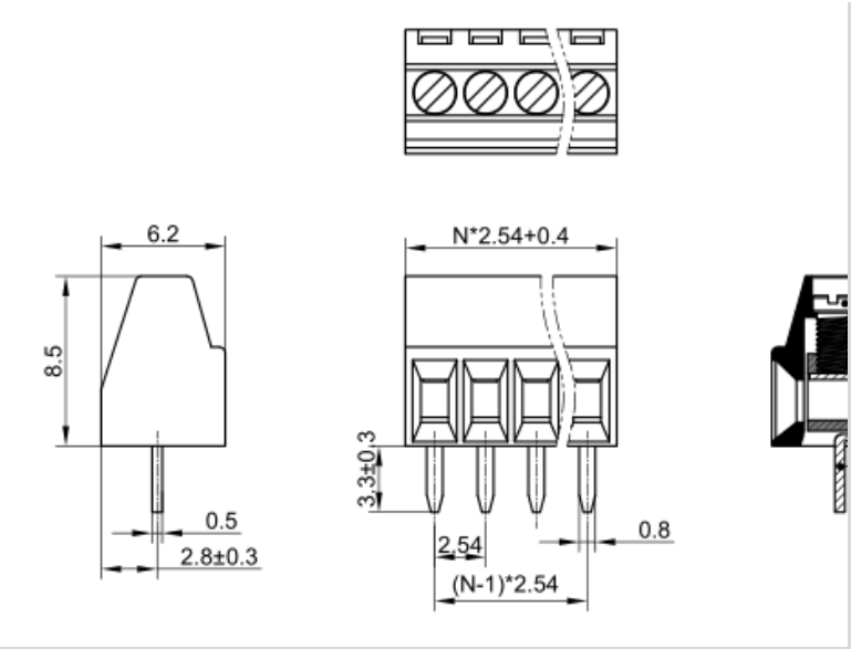
尺寸图
