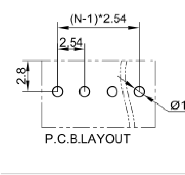
PCB 开孔图
